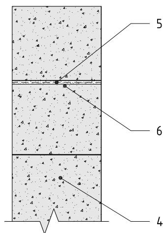
Pjūvis 1-1 Variantas 2 (armavimas tinkleliu)
