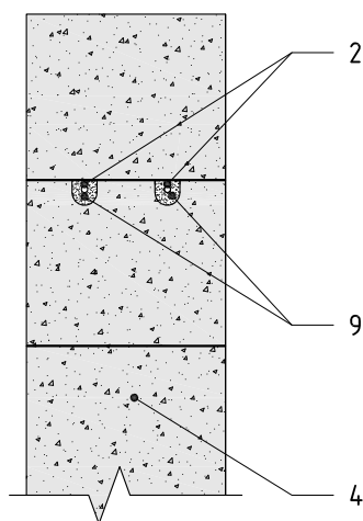
Pjūvis 1-1 Variantas 1 (armavimas formuojant išdrožas)
