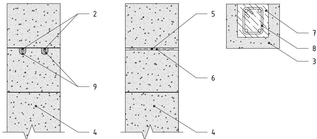
Pjūvis 1-1 Variantas 1 (armavimas formuojant išdrožas)
